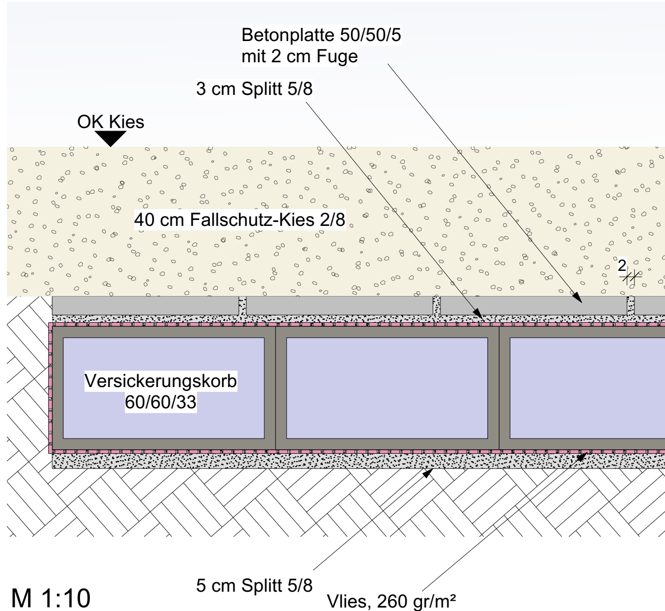
Detail: Versickerungskörbe unter Kiesfläche
