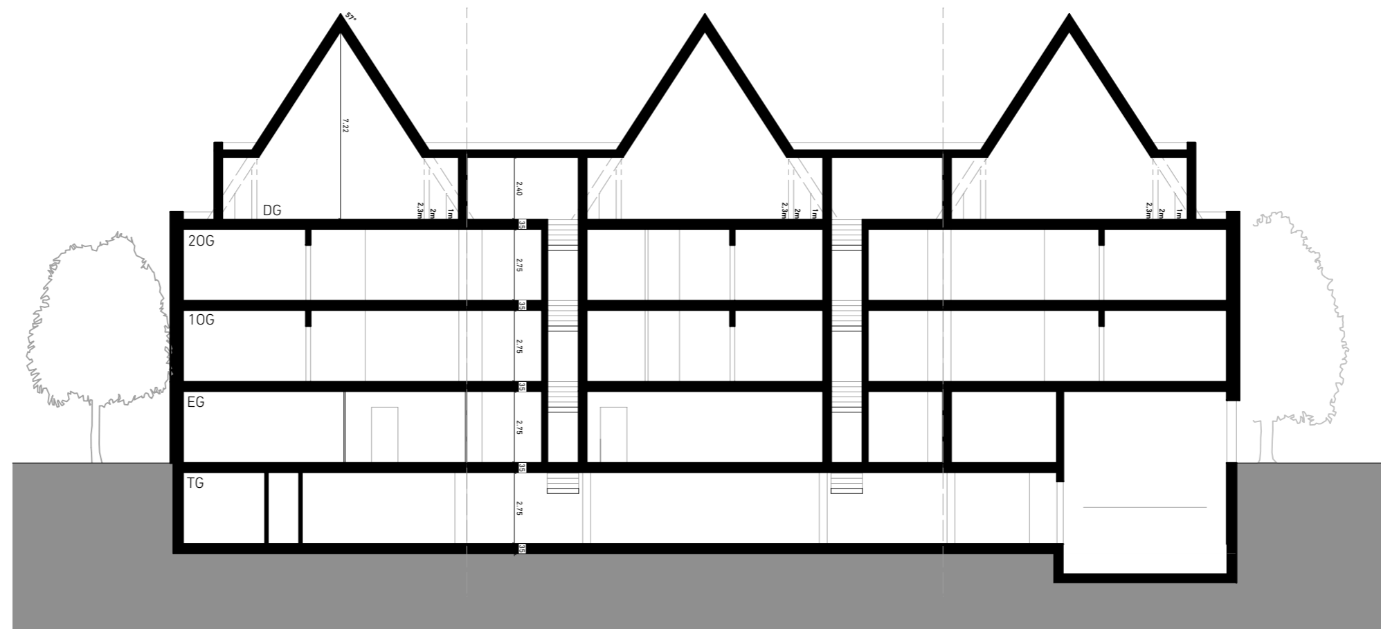
Schnitt B-B
