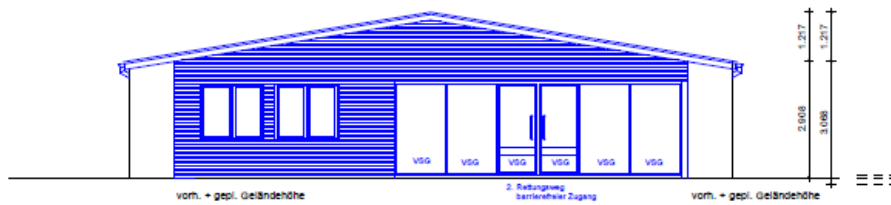
Ansicht Nord-West
