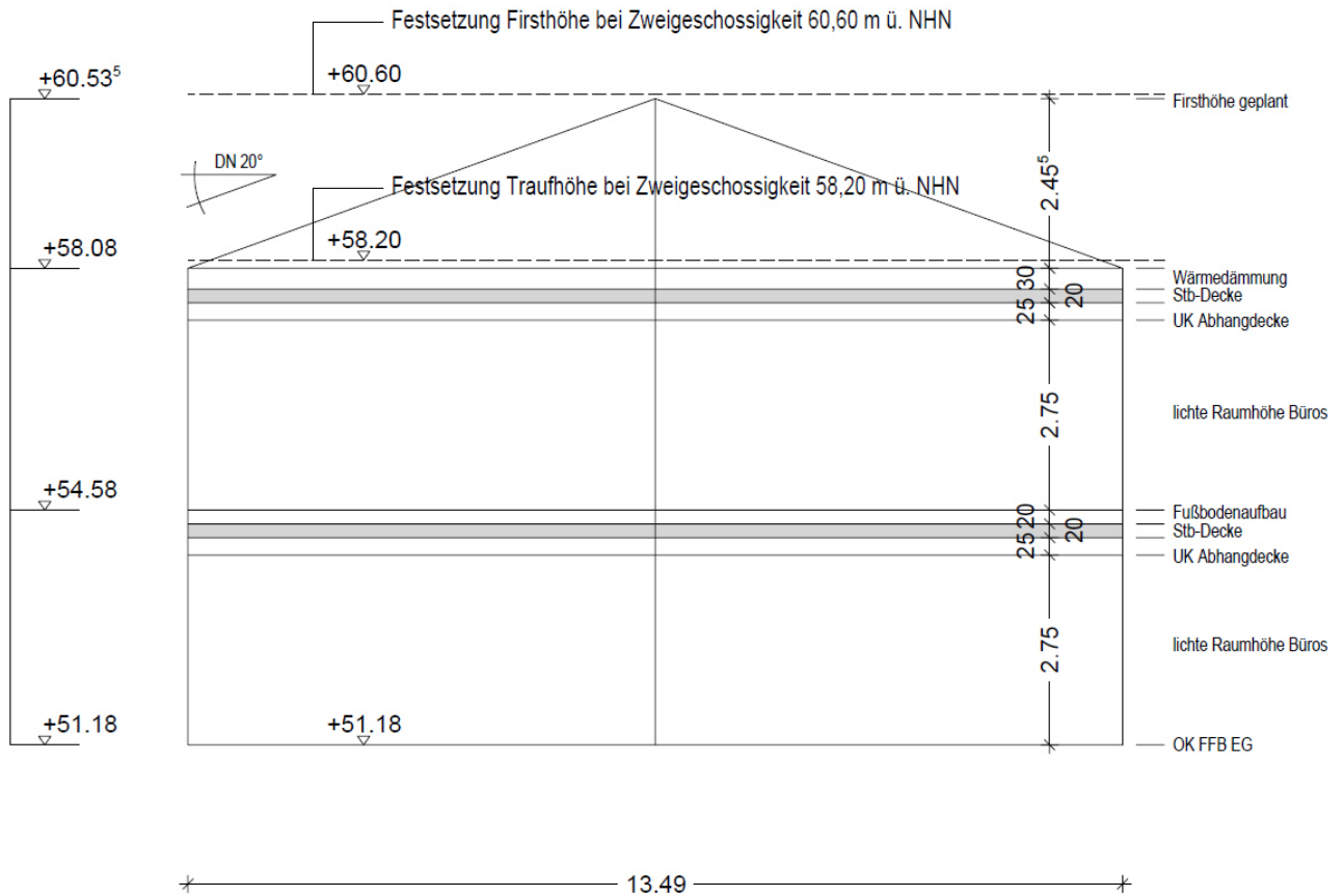
geplanter Erweiterungsbau zweigeschossig mit Satteldach DN 20°
