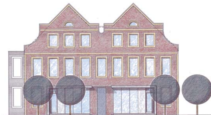
Ansicht Marktplatz
