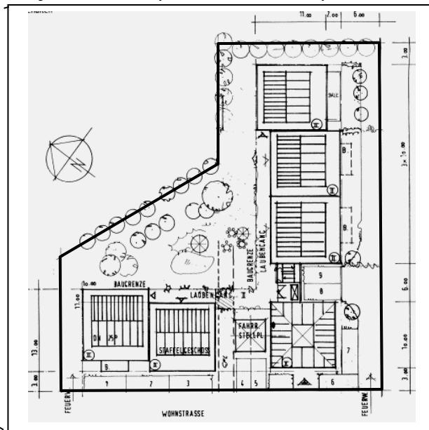
Projektentwurf (nicht maßstäblich)
