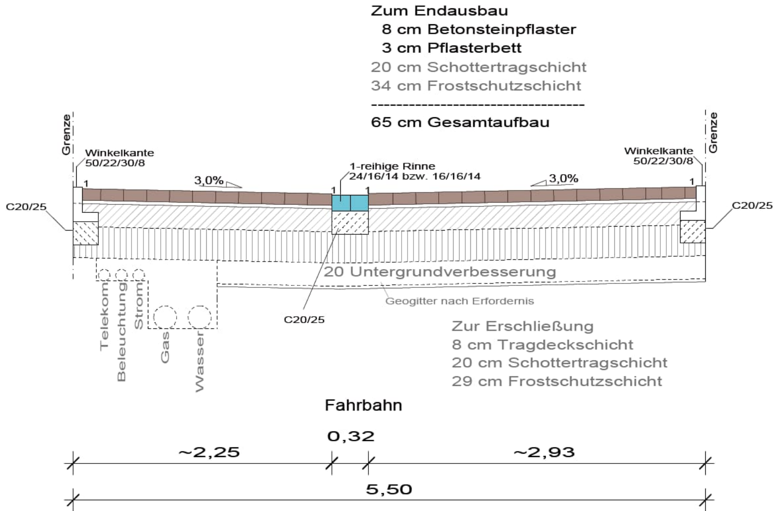
Regelquerschnitt 3
